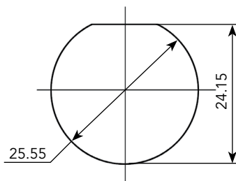
Jam Nut Receptacle - UTS7
