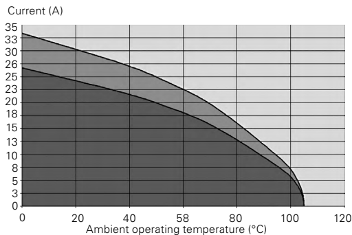
Fig.3: UTGX 12-4 – 2.5 mm 2 wires
